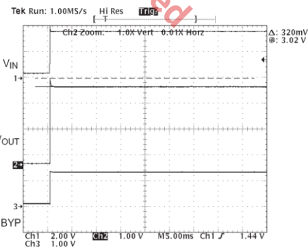
Fig. 15: Fast V_{IN} , No Load
